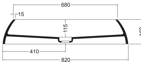
SEZIONE LONGITUDINALE LONGITUDINAL SECTION
