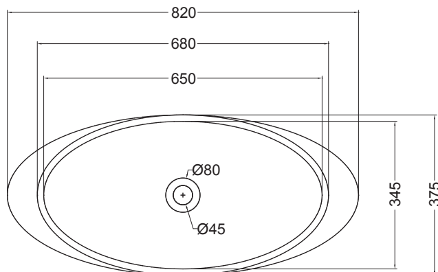
PIANTA PLAN
