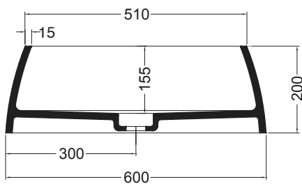
SEZIONE LONGITUDINALE LONGITUDINAL SECTION
