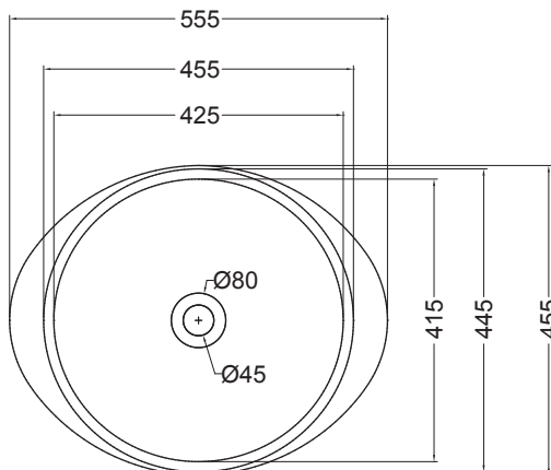
PIANTA PLAN
