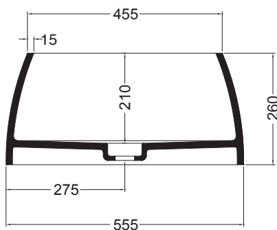
SEZIONE LONGITUDINALE LONGITUDINAL SECTION
