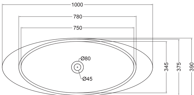
PIANTA PLAN
