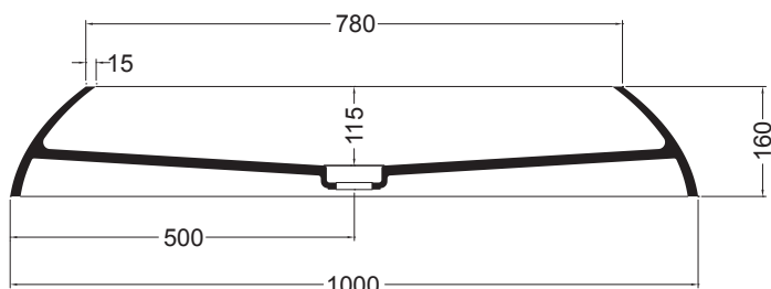
SEZIONE LONGITUDINALE LONGITUDINAL SECTION
