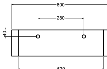
VISTA POSTERIORE
