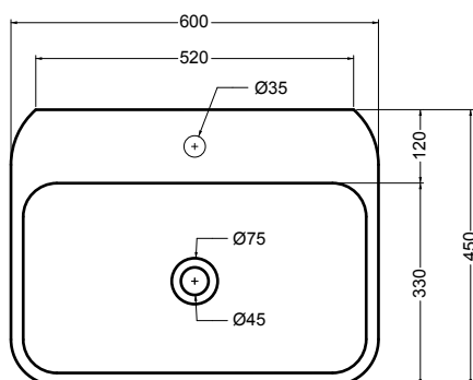
PIANTA
