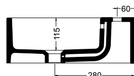
SEZIONE TRASVERSALE
