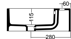
SEZIONE TRASVERSALE CROSS VIEW
